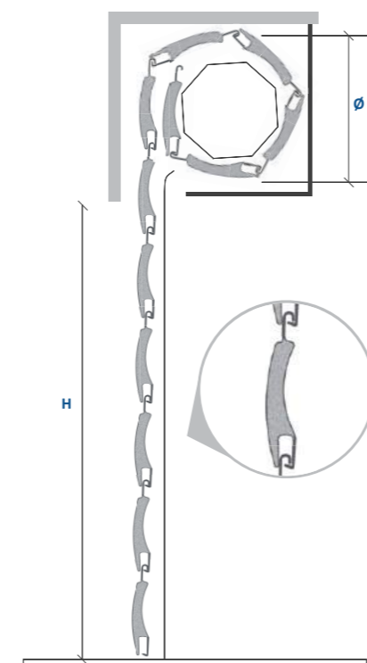
H= MISURE LUCE Ø= DIAMETRO DI AVVOLGIMENTO SU RULLO
